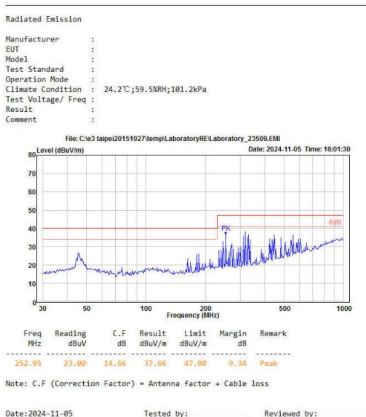
图 5-7 辐射测试垂直方向
